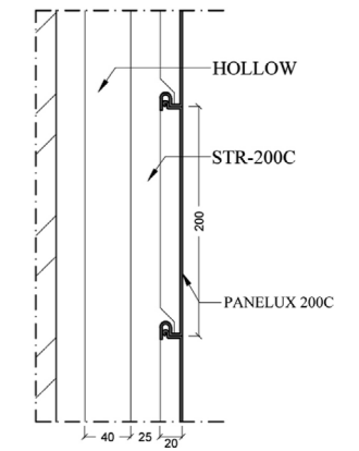
DETAIL-A SKALA 1:5
