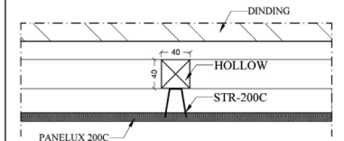
DETAIL-B SKALA 1:5
