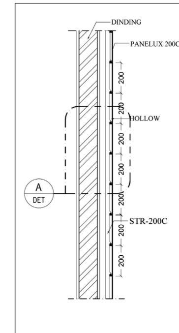
POTONGAN-A SKALA 1:5
