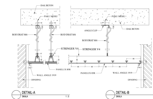
LINEAR CEILING 85R V4
